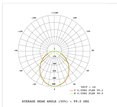
Courbe 30W - 3000K
