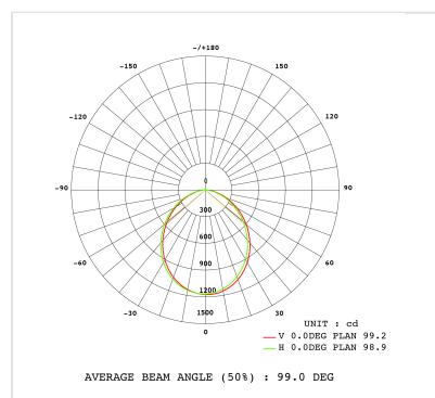
Courbe 30W - 4000K
