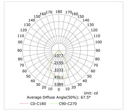
Courbe 4000K
