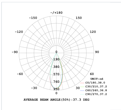
Courbe 6W 3000K
