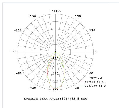
Courbe 8W_2700K
