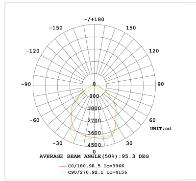
Courbe 5000K
