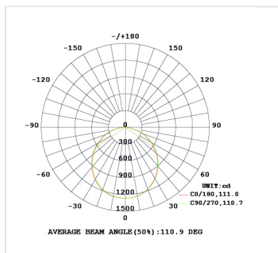
Courbe 36W - 2700K
