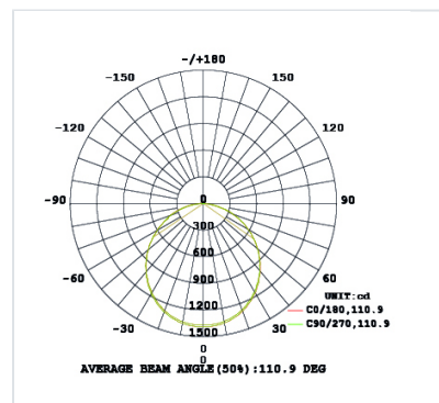
Courbe 36W - 4000K
