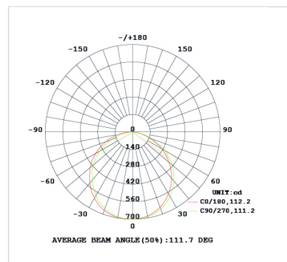
Courbe 20W - 4000K
