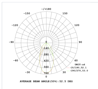
Courbe 8W_2700K
